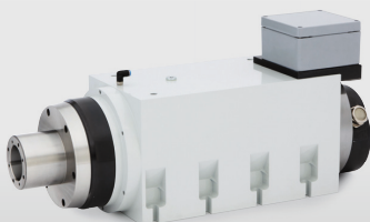
Motorkastenspindeln Motor box spindles
